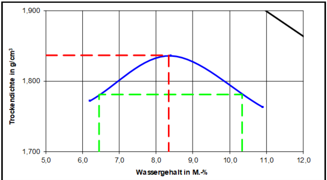
Proctorkurve des untersuchten RC-Materials 0/45 (aus Prüfbericht F 18/05/0359– II/2018)
