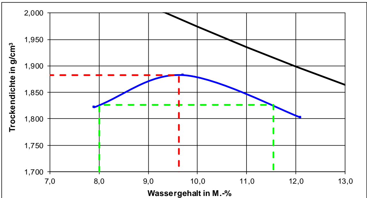
Proctorkurve der untersuchten RC 0/11 (aus Prüfbericht Nr. F 18/11/1018)
