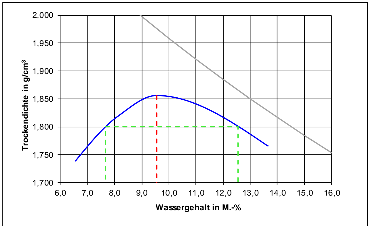
Proctorkurve des untersuchten RC-Materials 0/45
