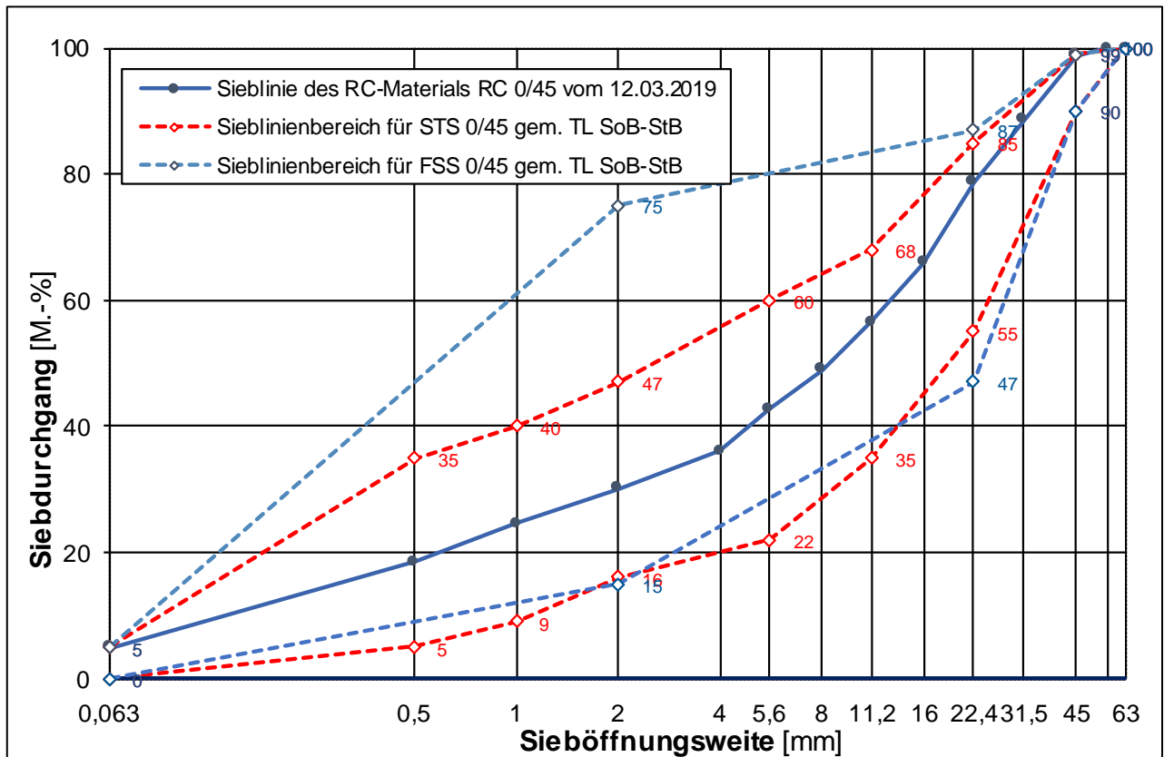
Korngrößenverteilung des untersuchten RC-Materials 0/45 mit Sieblinienbereich für Schottertrag- und Frostschutzschichten 0/45 mm gemäß TL SoB-StB /8/
