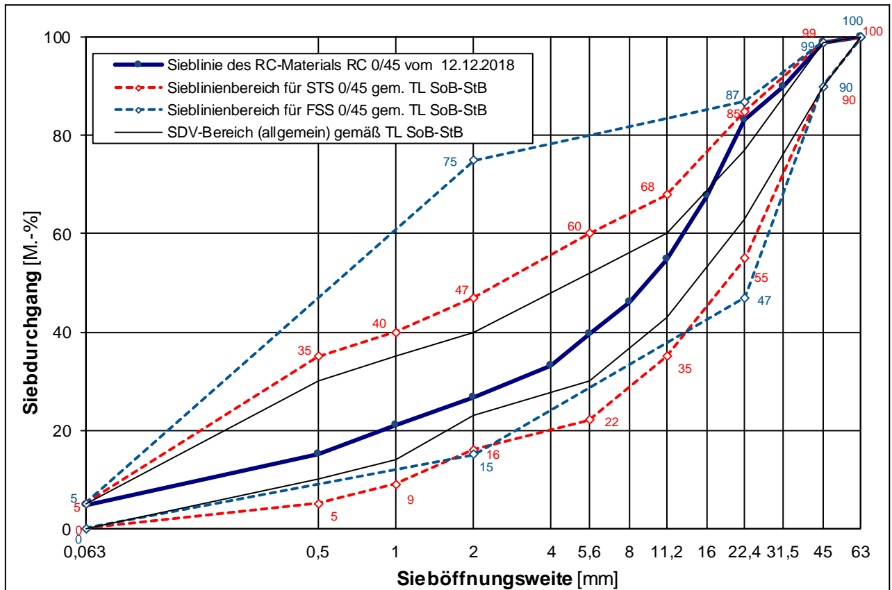
Korngrößenverteilung des untersuchten RC-Materials 0/45 mit Sieblinienbereich für Schottertragschichten 0/45 mm gemäß TL SoB-StB /8/
